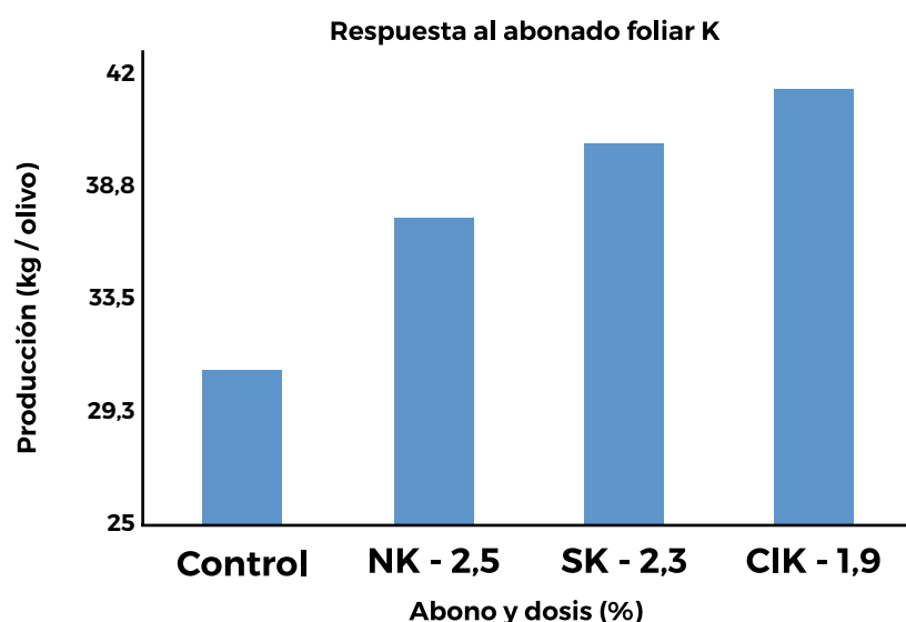
Figura 4. Respuesta del olivar de riego a aportaciones foliares con diferentes abonos potásicos.
